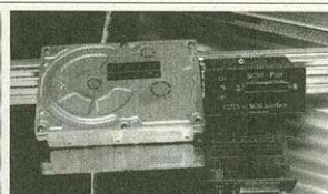
CDTV to SCSI Interface Ihr CDTV Harddisk Controller 16 Mhz Turbotakt, HD's intern oder extern.
